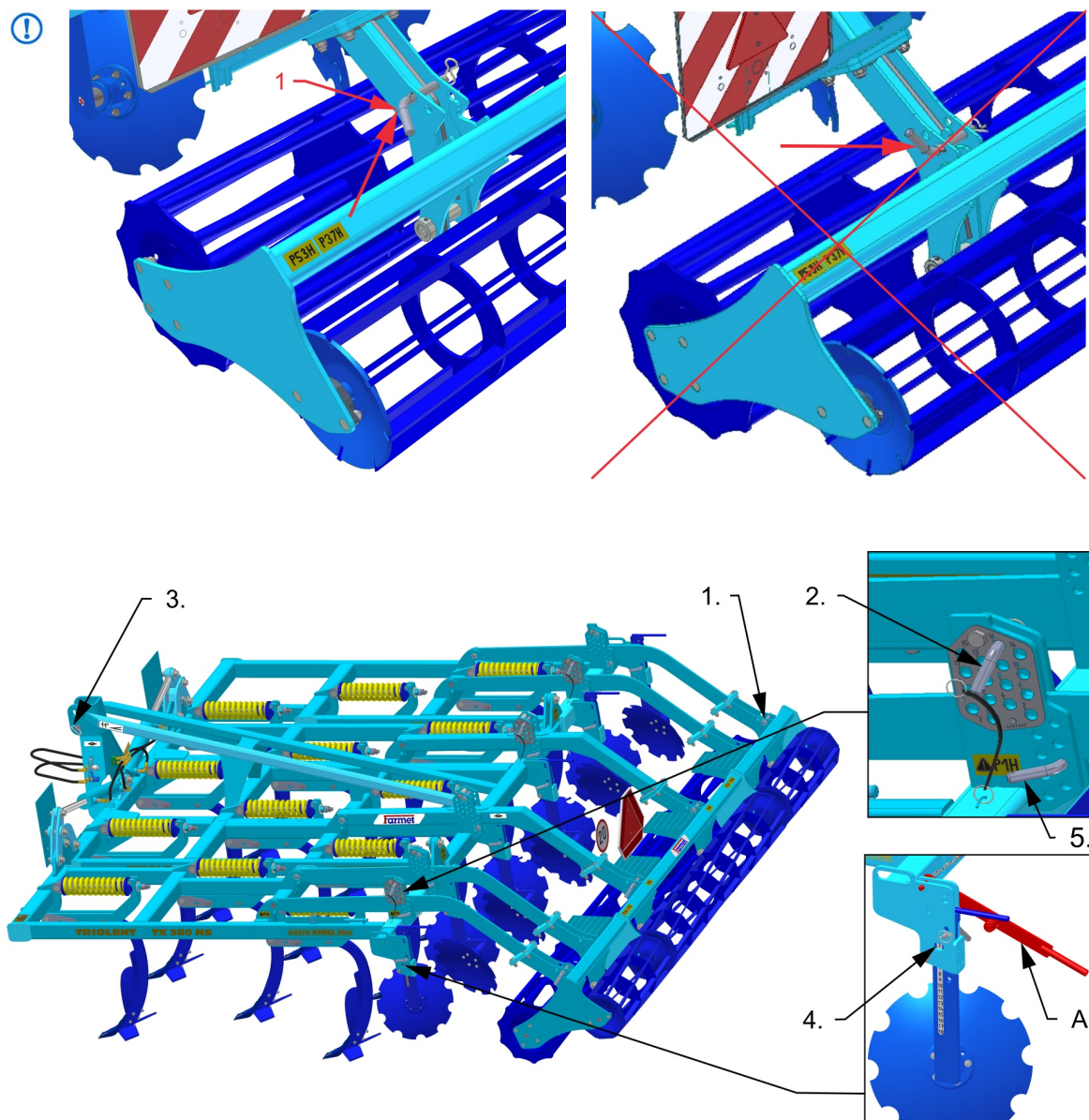
Obr. 7 - postup seřízení stroje
