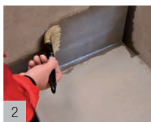
Penetrovat podklad - sjednotit savost.
