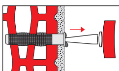
Krok 7 - Nadávkovat do otvoru maltu. Otvor zcela vyplnit kotevní maltou. Při vsunutí kotvicího prvku dojde k vytlačení kotvicí malty skrze sítko do dutin v cihle.
