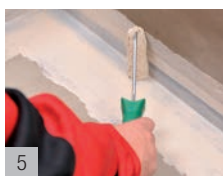
Vtlačit válečkem Těsnicí pásy do svislých a vodorovných koutů.
