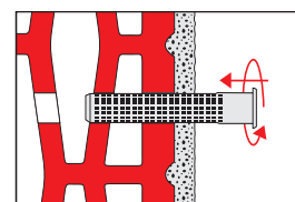
Krok 5 - Vsunut do vyvrtaných otvorů sítko.
