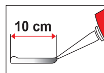
Krok 6 - Nasadit kartuši do pistole, našroubovat mísicí trysku. Vytlačit asi 10 cm kotevní malty mimo připravené otvory, dokud není dosaženo rovnoměrné šedé barvy.
