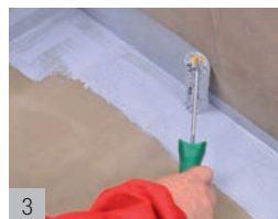
3 Nanést hydroizolaci na exponovaná místa.
