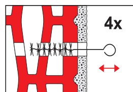
Krok 3 - Uvolnit nesoudržný prach pomocí kartáčku.
