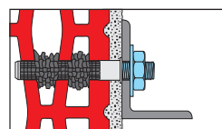
Krok 8 - Vsunut do otvoru kotvený prvek otáčivým pohybem ve směru závitu – prvek tzv. zašroubovat.
