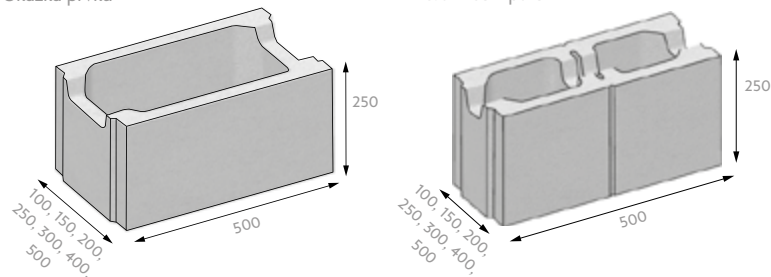
Ukázka prvku
