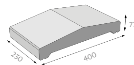
stříška 30 štípaná
