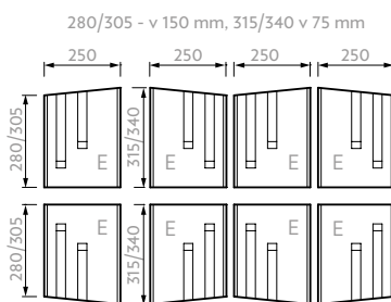
NATURBLOK ROH
