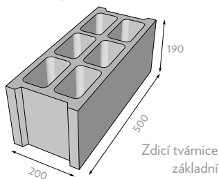
Ukázka prvku
