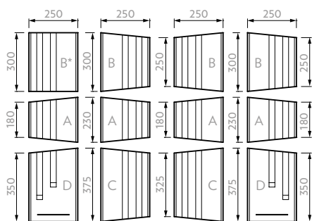
NATURBLOK kámen
