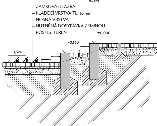
řez a-a'
