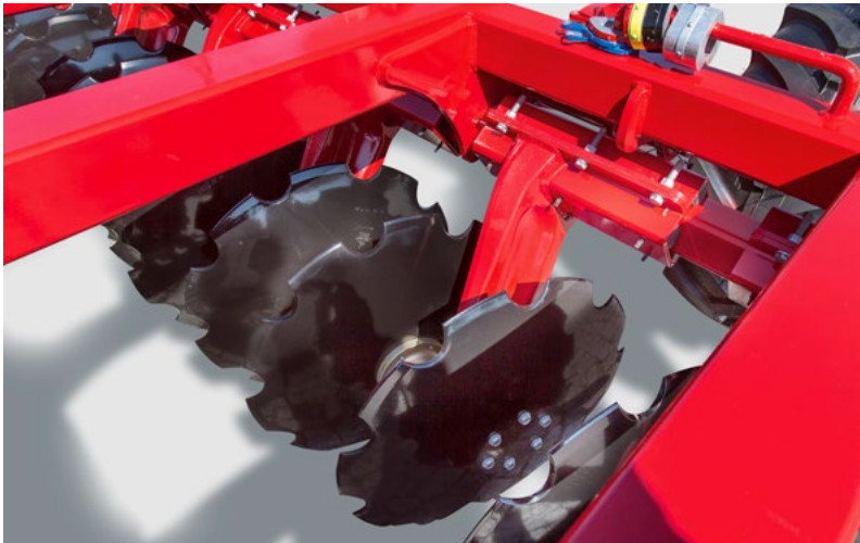
Velké talíře (Ø 62 cm) pro hlubokou práci
