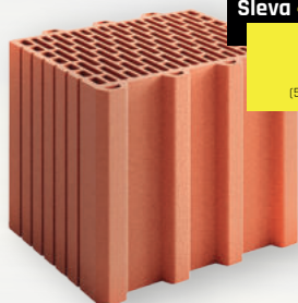
LEIERPLAN 30 N+F P10 Rozměr: 300 x 250 x 249 mm
