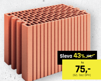
LEIERPLAN 25 N+F P10 ✓ Rozměr: 250 x 375 x 249 mm
