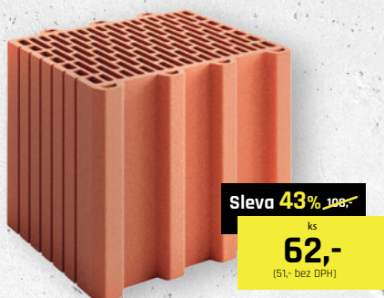
LEIERPLAN 30 N+F P10 ✓ Rozměr: 300 x 250 x 249 mm
