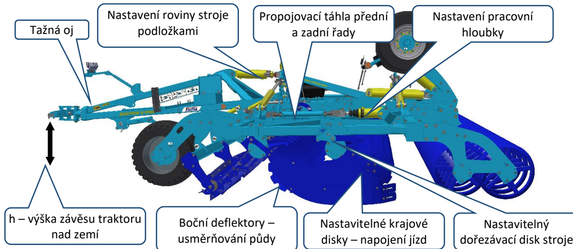
Obrázek 13 Seřízení stroje
