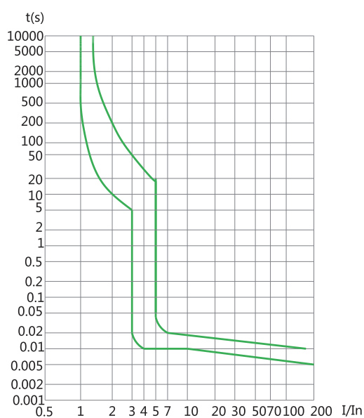
Caracteristica B
