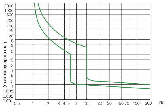
Caracteristica C
