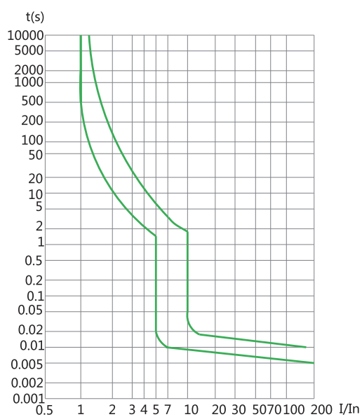
Caracteristica C
