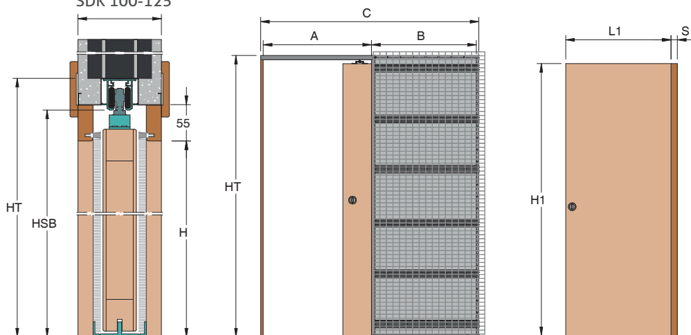
ZEĎ 90-107-125-145 SDK 100-125
