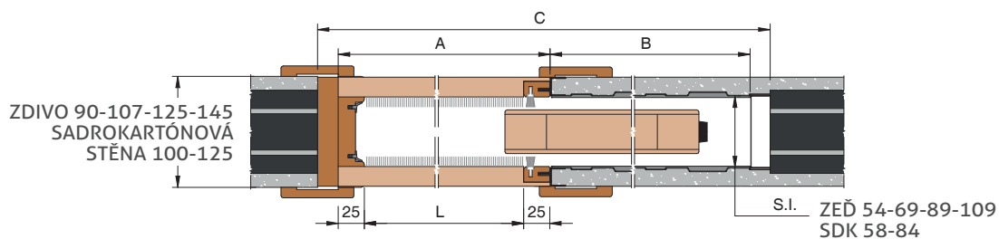
ZEĎ 90-107-125-145 SDK 100-125
