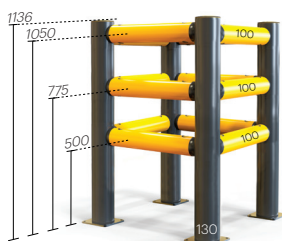
iFlexRail Ochrana sloupů Column Guard ***
