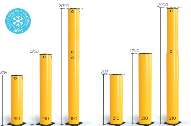
iFlex Bollard s dvojitým otočným opláštěním ***
