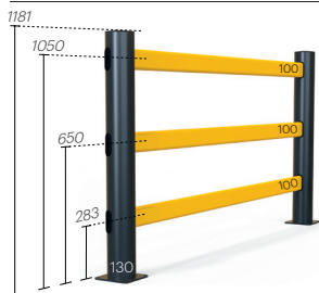
eFlex Pedestrian Barrier 3tyčová *
