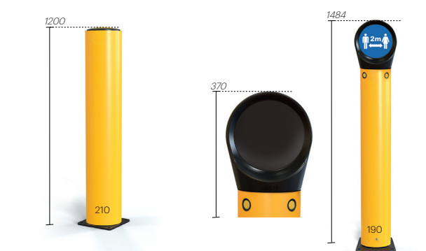
iFlex Bollard s dvojitým otočným opláštěním ***
