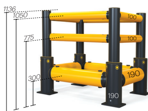
iFlexRail Ochrana sloupů Column Guard+ ***
