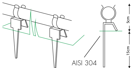
90106008 Coppia picchetti INOX - Orizzontale Couple INOX stakes for fied - horizontal Paar INOX Pflöcke für Rasen - horizontal
