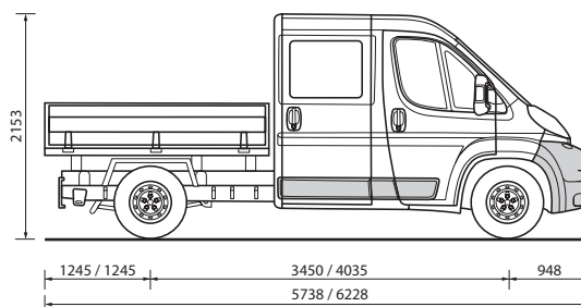
Valník Dvoubabina
